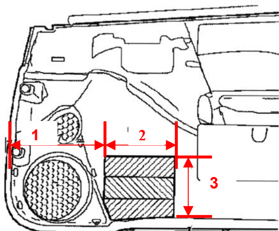
Binnenaanzicht portierbekleding
