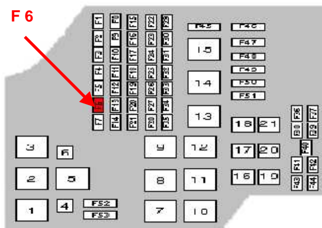
sikringsboks motorrum
