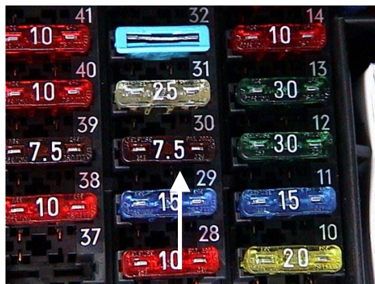
Fig. 2 Sikring 30
