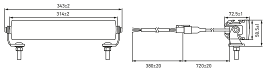
Met zijmontagebeugel
