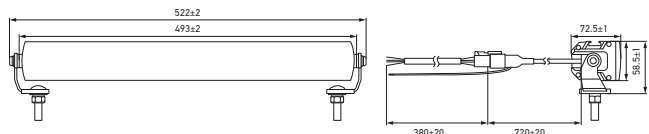
Met zijmontagebeugel
