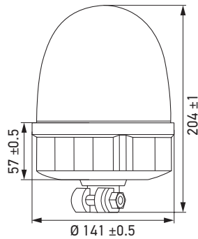
Versie met flexibele buismontage
