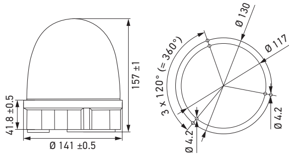
Versie met vaste montage
