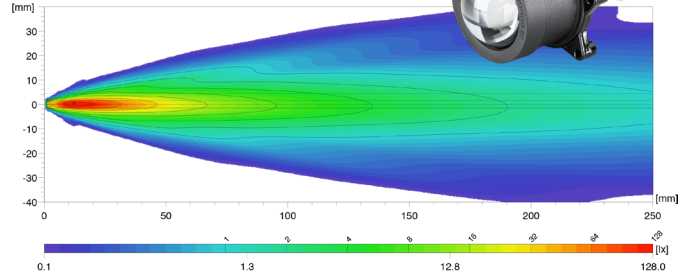
Module 60 Halogen (R149 Class DS) (998 570)
